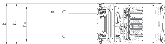
Vista superior
