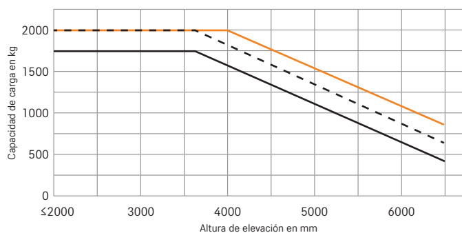
RCE 20P Mástil triple 4800 mm - ruedas SE
