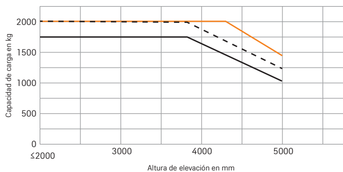
RCE 20 Mástil triple 4800 mm - ruedas SE
